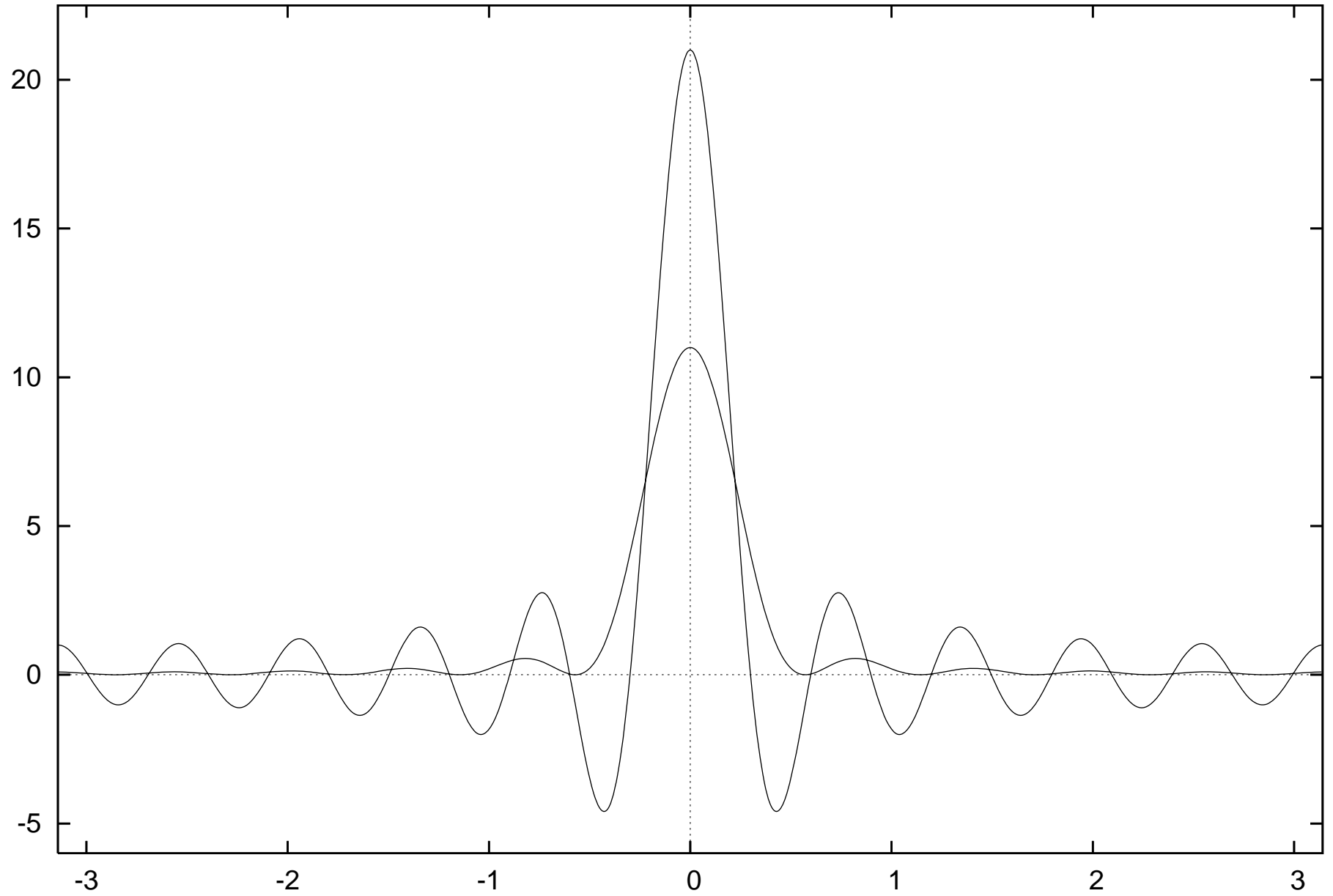
Dirichletkern und Fejerkern, n=10
