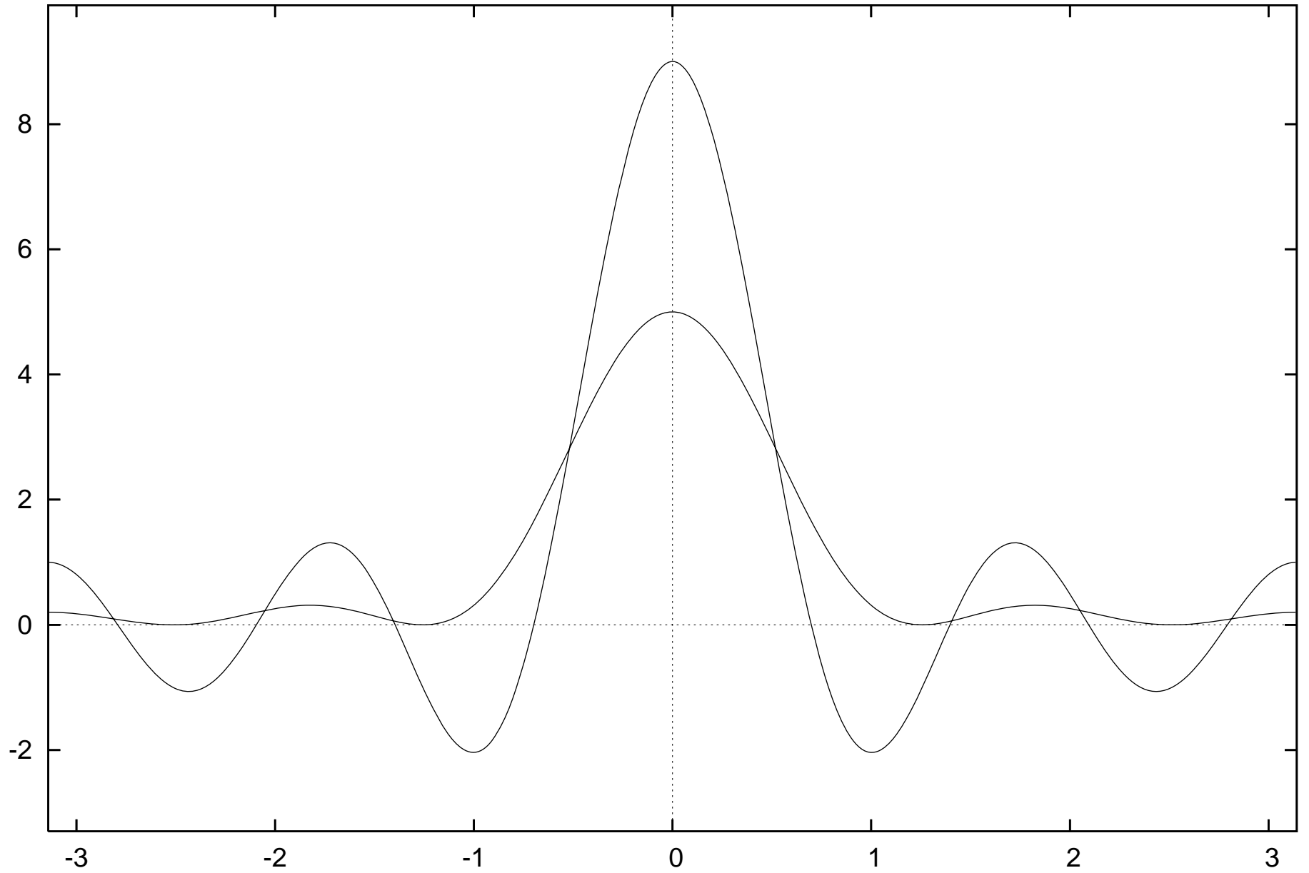
Dirichletkern und Fejerkern, n=4
