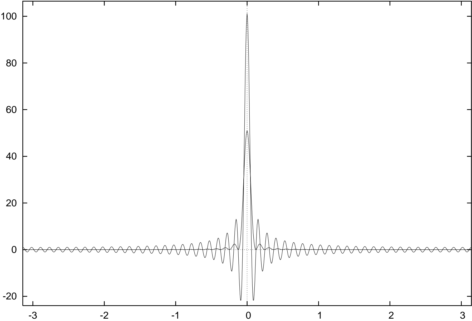
Dirichletkern und Fejerkern, n=50
