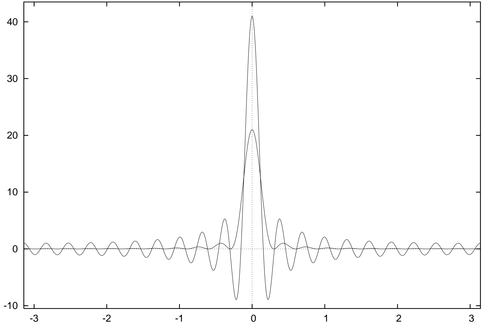
Dirichletkern und Fejerkern, n=20
