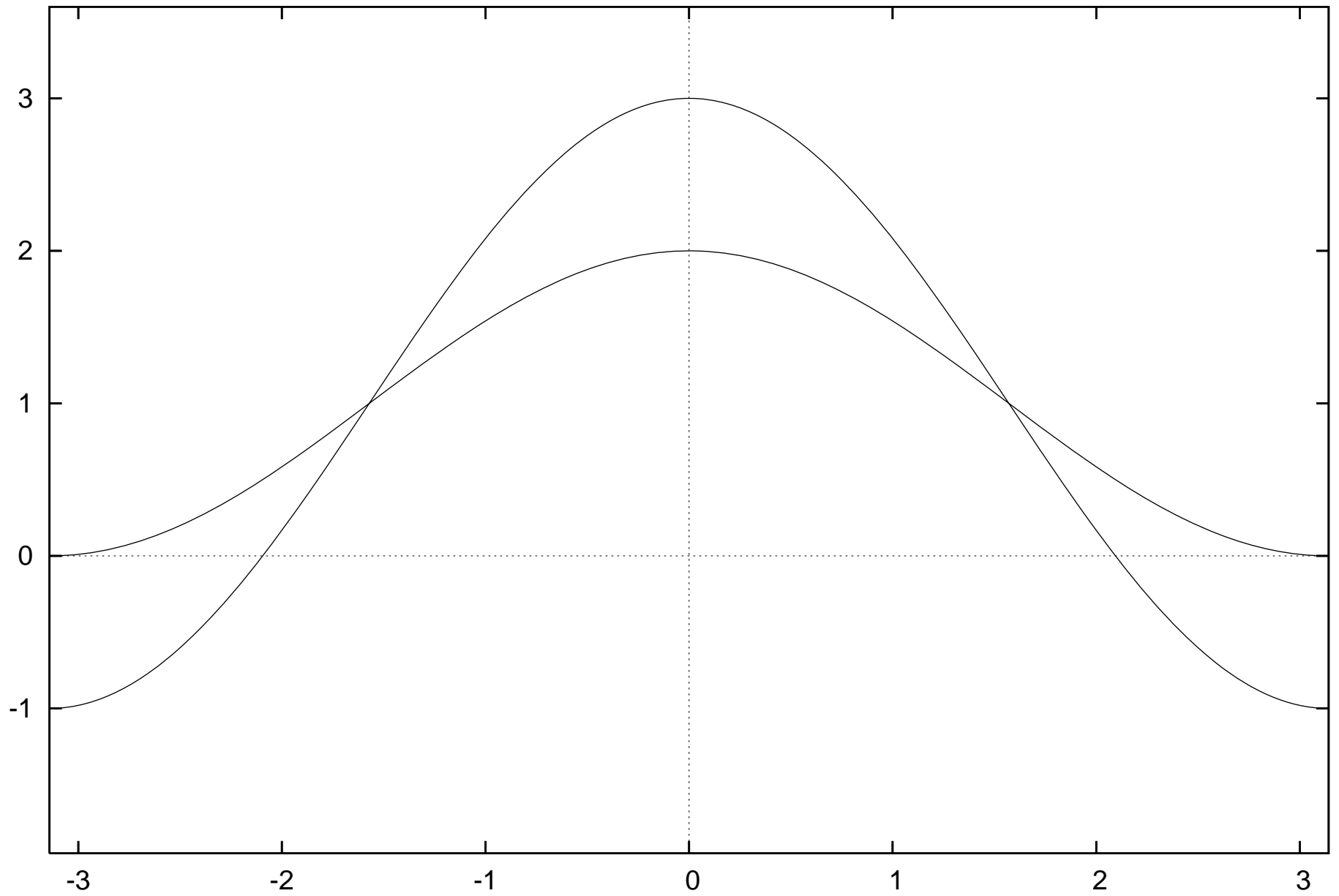
Dirichletkern und Fejerkern, n=1
