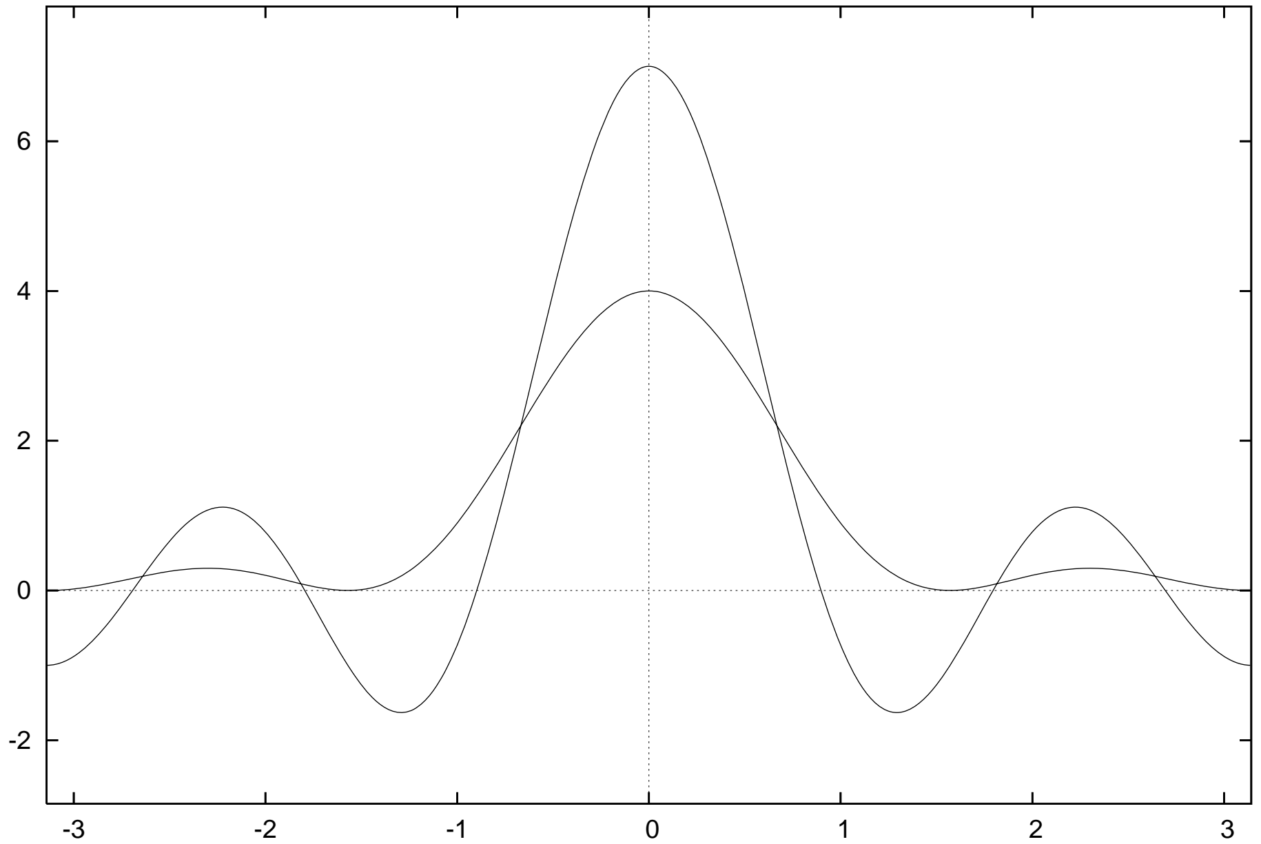
Dirichletkern und Fejerkern, n=3
