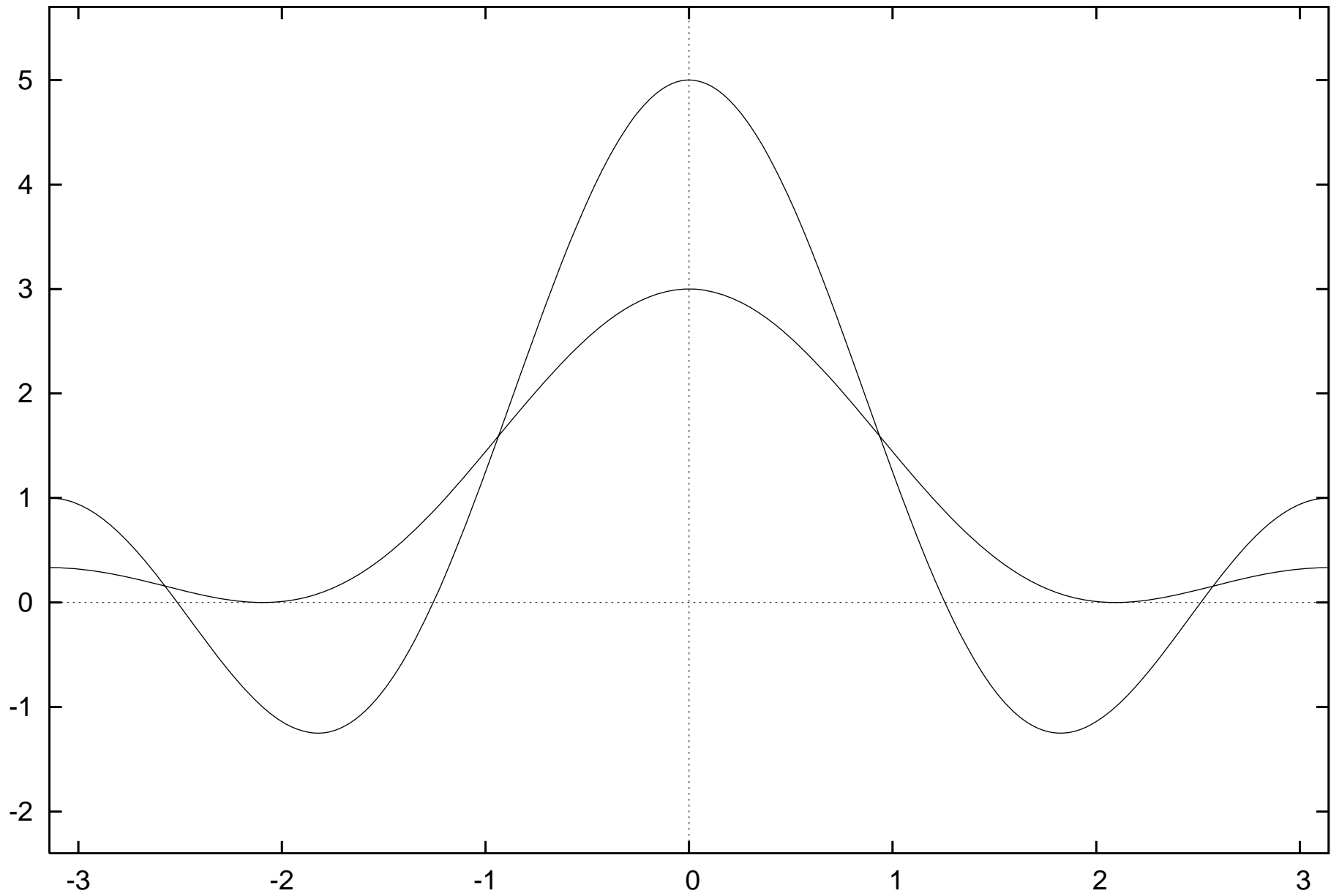
Dirichletkern und Fejerkern, n=2
