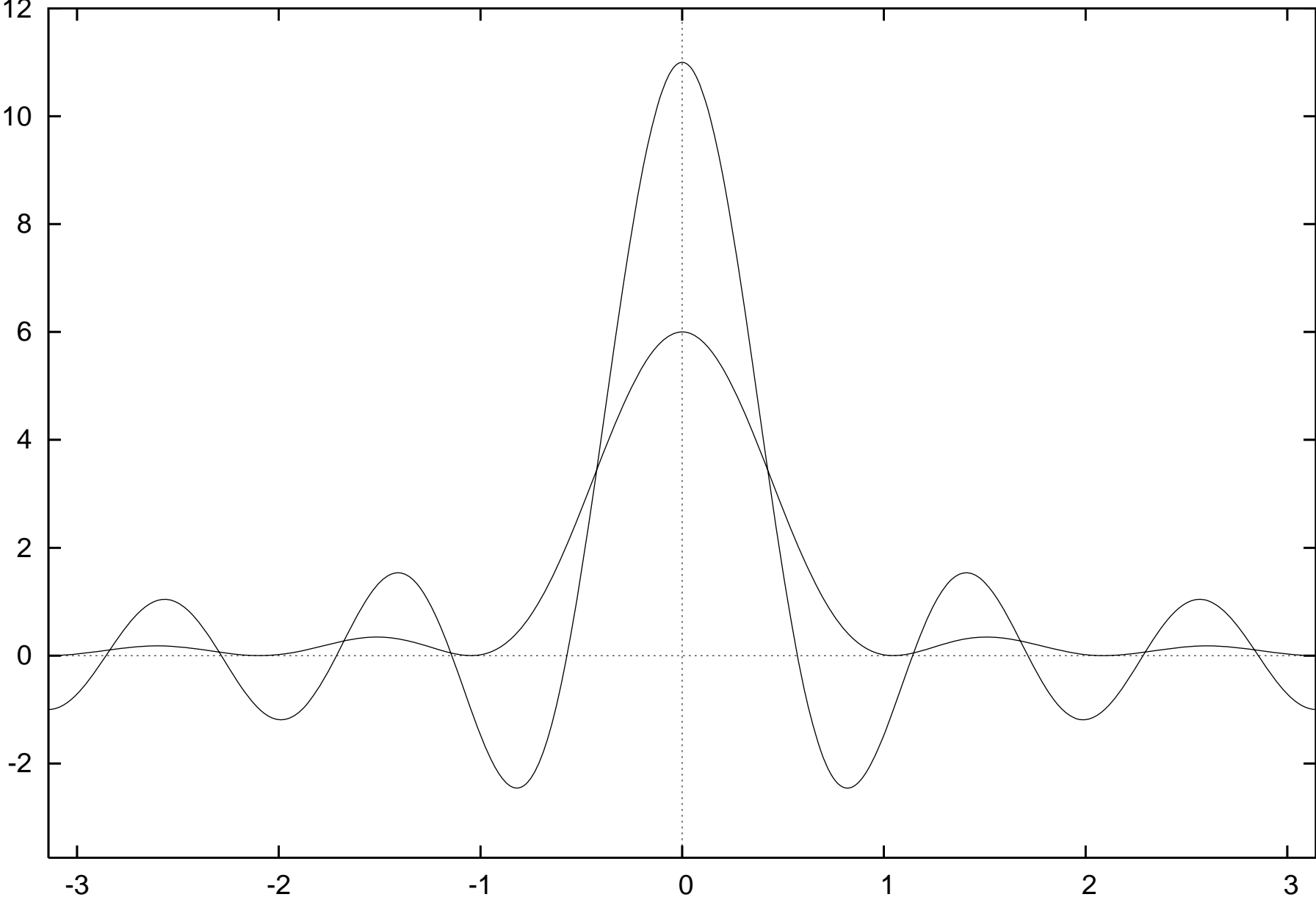
Dirichletkern und Fejerkern, n=5
