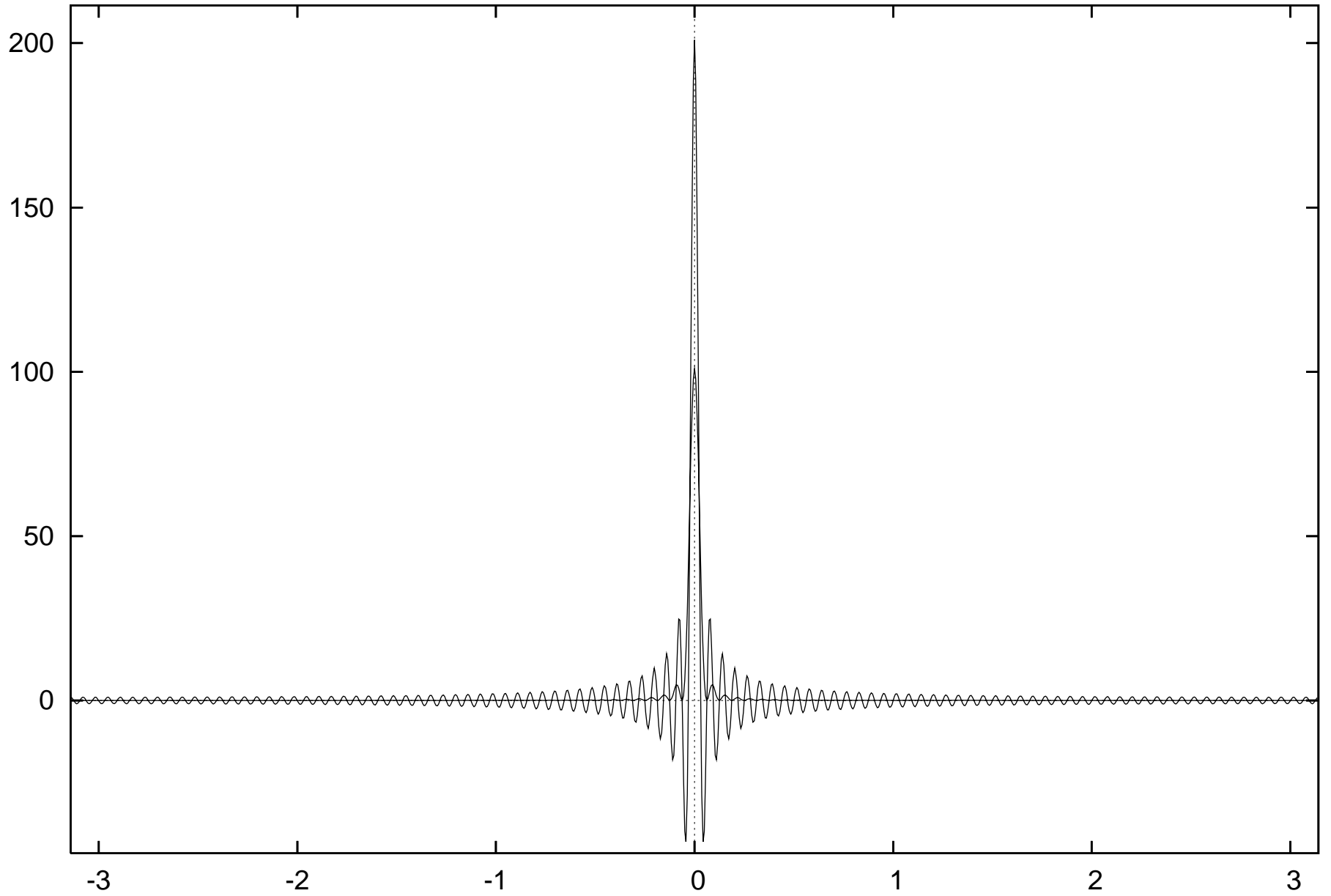
Dirichletkern und Fejerkern, n=100
